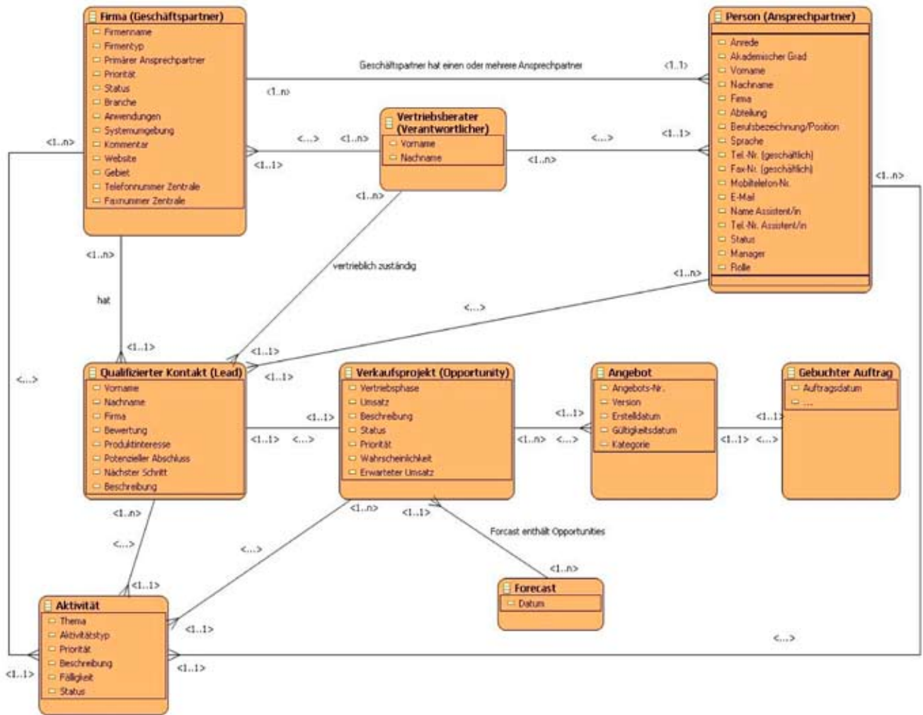
Abbildung 3: Objektmodell (Datenbankstrukturen)
